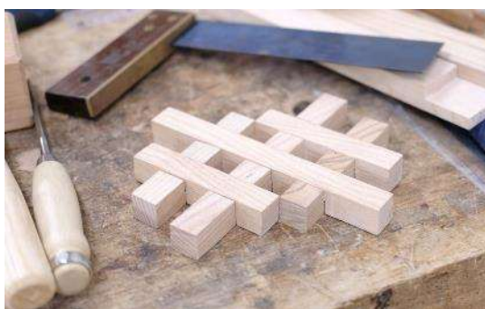
Enchevêtrement de mi-bois
