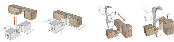
Croix du charpentier
